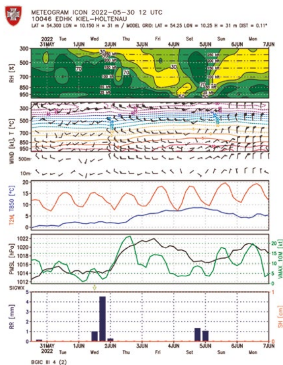
△ Abb. 1a: Meteogramm für den Standort Kiel-Holtenau basierend auf dem ICON-Modell vom 30. Mai 2022, 12 UTC. (Quelle: Bundeswehr/ZGeoBw/Holz hacker & Zygmuntowski)
