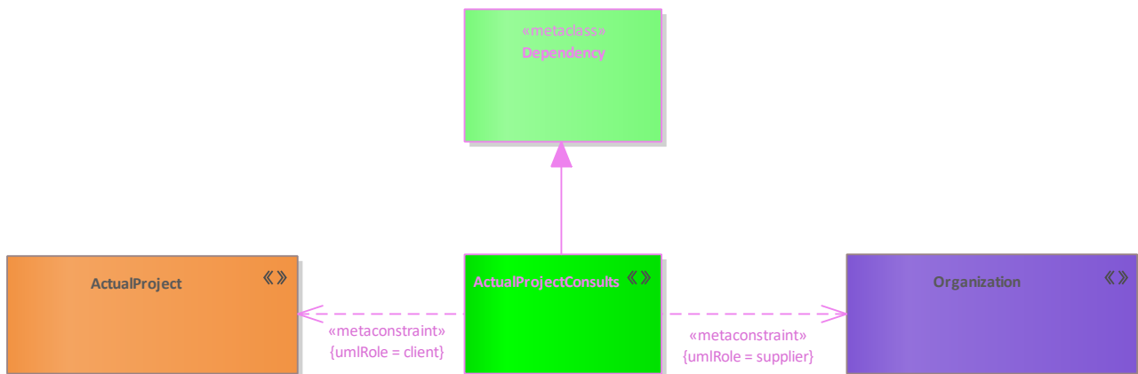
Figure 77: ActualProjectConsults
