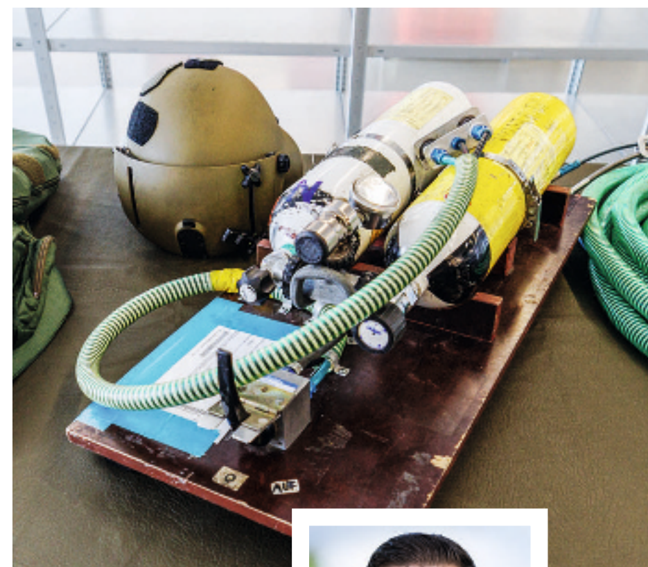
Ohne Druckluft geht nichts Der Feuerlöschbehälter wird mit Druckluft geschlossen und geöffnet. Die Druckluftflaschen werden vor jedem Flug kontrolliert.
